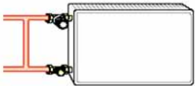
RADIAATOR KOOS HEIMEIERI VÄIKESETAKISTUSELISE TERMOSTAATVENTIILI, TERMOPEA K JA SULGEVENTIILIGA REGUTEC
