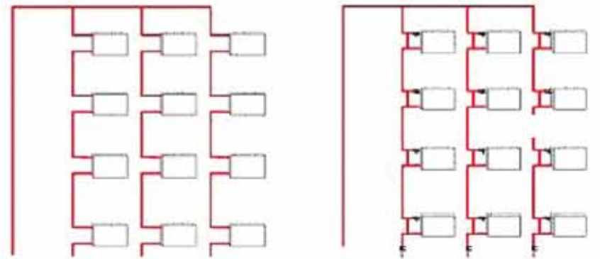
JOONIS 2. MÖÖDAVIIKUDETA ÜHETORUSÜSTEEMI RENOVEERIMINE
