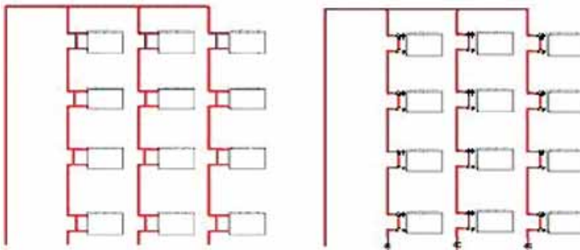
JOONIS 3. MÖÖDAVIIKUDEGA ÜHETORUSÜSTEEMI RENOVEERIMINE 3T-TERMOSTAATVENTIILIDE ABIL
