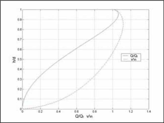
JOONIS 4. QMAX-TORUDE LÄBILASKEVÕIME Q JA VOOLUKIIRUSE v OLENEVUS SUHTELISEST TÄISTEST h/d ( h ON TÄIDE JA d TORU SISEKÕRGUS; Q_t JA v_t – VOOLUHULK JA KIIIRUS TÄISTÄITE PUHUL)
