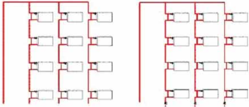
JOONIS 1. MÖÖDAVIIKUDEGA ÜHETORUSÜSTEEMI RENOVEERIMINE
