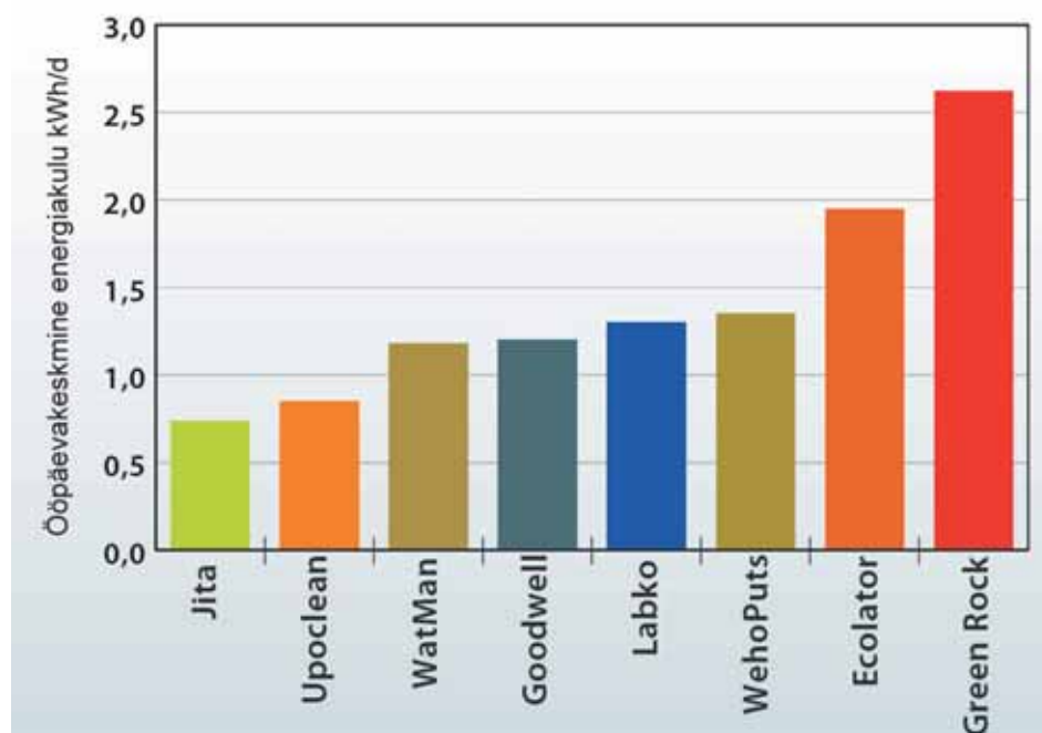
Joonis 2. Katsetatud puhastite ööpäevakeskmine energiatarve [2]
