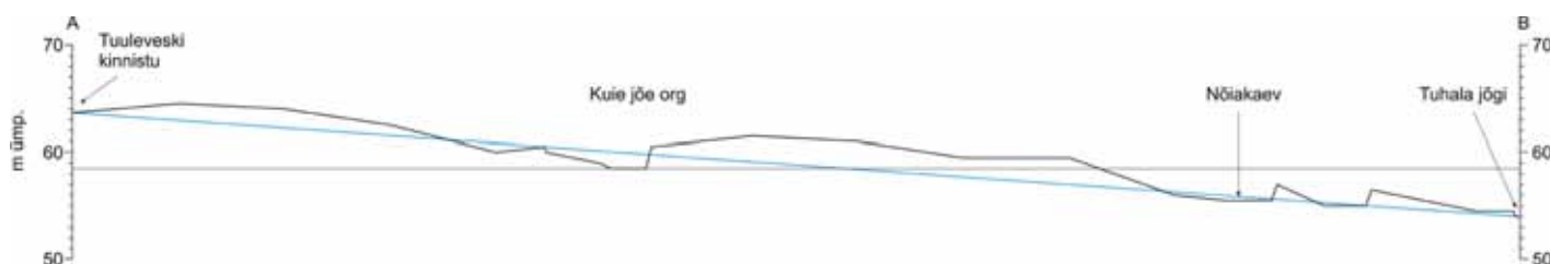
Joonis 3. Maapinna kõrgus ja põhjavee tase Tuuleveski kinnistu (A) ja Nõia-kaevu (B) vahelist joont mööda (vt joonis 2). Püstmõõtkava on 10 korda rõhtmõõtkavast suurem
