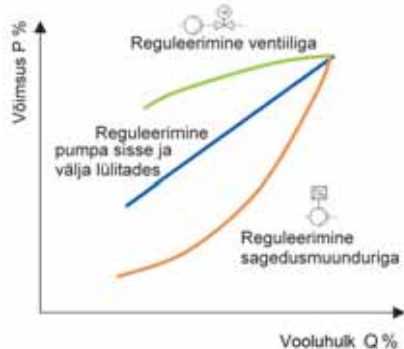
Pumba võimsustarbekõverad P(Q)
