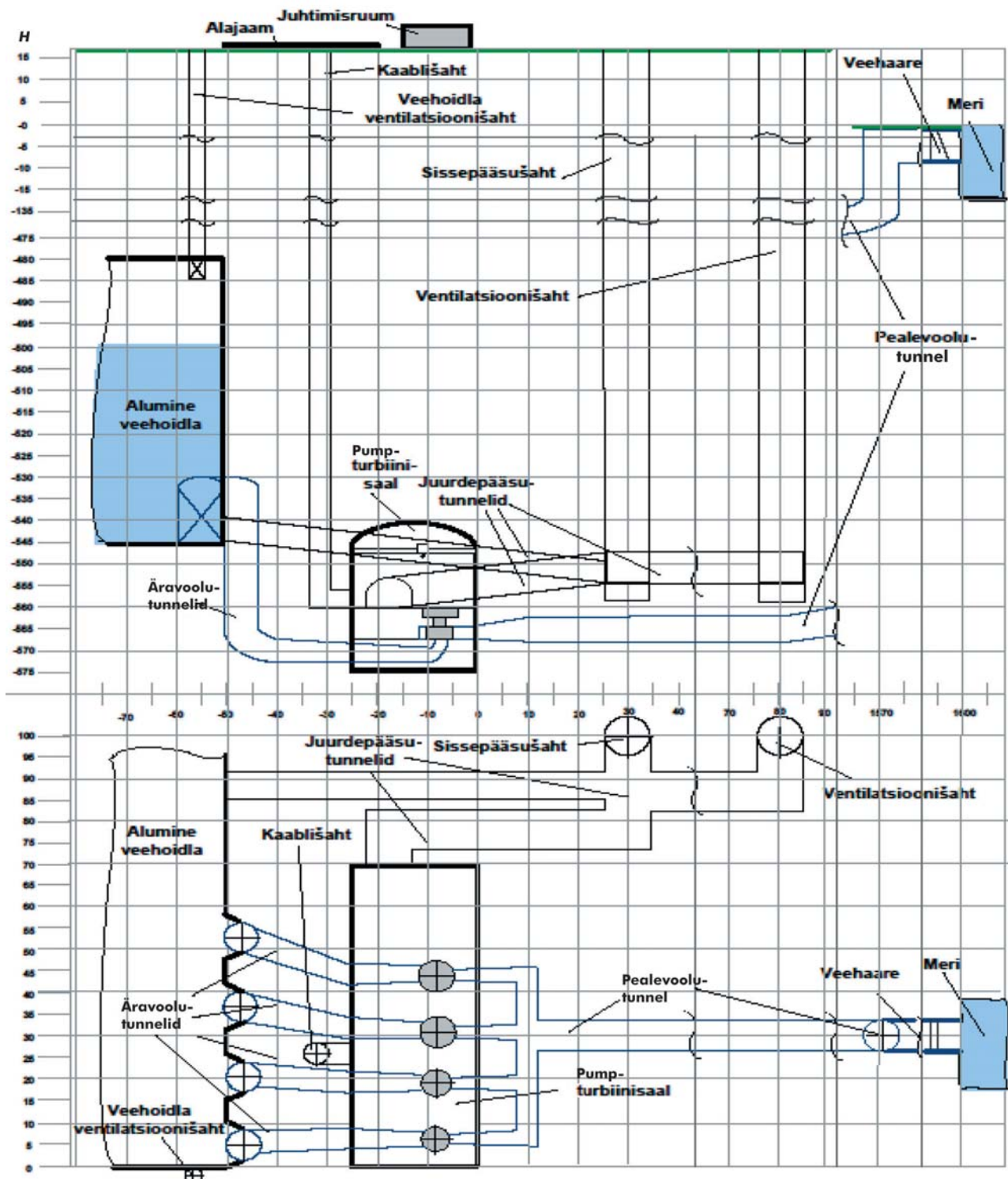
▲ Joonis 2. Kavandatav maa-alune pumpe-hüdroelektrijaam. Pumpamisrežiimis muutuvad äravoolutunnelid pumpturbiinide imitorudeks ning pealevoolutunnel survetoruks
