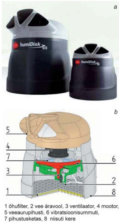
Joonis 1. Õhu tsentrifugaalniisuti humiDisk: a niisutid jõudlusega 6,5 ja 1 kg vett tunnis, b õhuniisuti lõige
