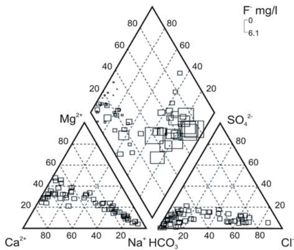
Joonis 3. Piperi diagammid iseloomustavad S–O veeladestu põhjavee F- ja B-sisaldust sõltuvalt vee keemilisest tüübist
