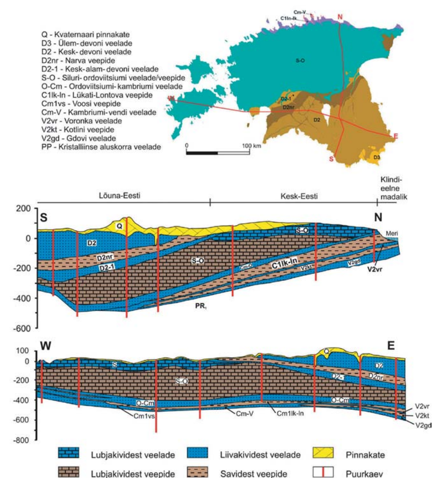
Joonis 3. Veejuhtivusest sõltuvalt jagunevad Eesti aluspõhjakivimid veelademeteks ja veepidemeteks. Läbilõigete asukohad on üllemisel skeemil näidatud punaste joontega
