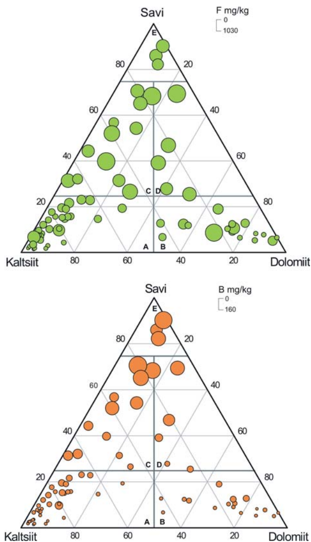
Joonis 4. Kivimiproovide F- ja B-sisaldus sõltuvalt kivimitüübist. Karbonaatkivimite klassifikatsioon ainelise koostise järgi ([10] põhjal):
