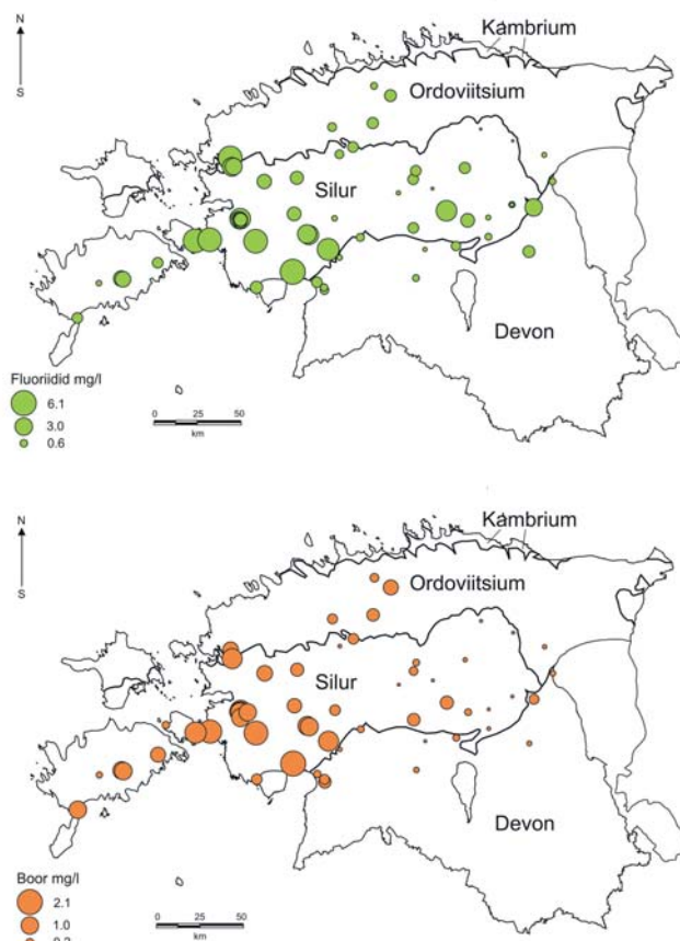
Joonis 1. F- ja B levik ning sisaldus S-O veeladestus
