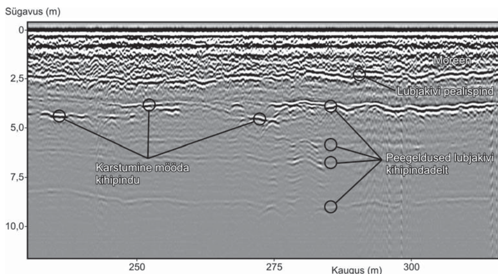
Georadar võimaldab määrata pinnakatte paksust ja karstinähtuste iseloomu. Joonisel on näha kihipindu mööda arenenud karstumine Pandivere kõrgustikul
