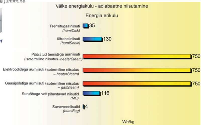
Joonis 4. Õhuniisutite energia erikulu Wh kg vee kohta
