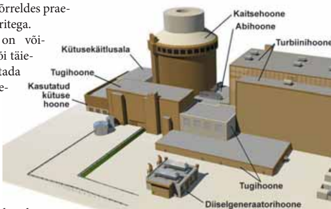
Joonis 1. Tuumareaktor Westinghouse AP1000™ Allikas: www.ap1000.com
