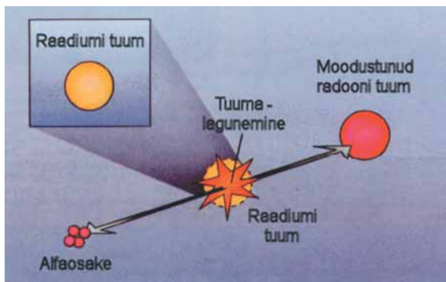
Joonis 1. Ra-226 tuuma lagunemine
