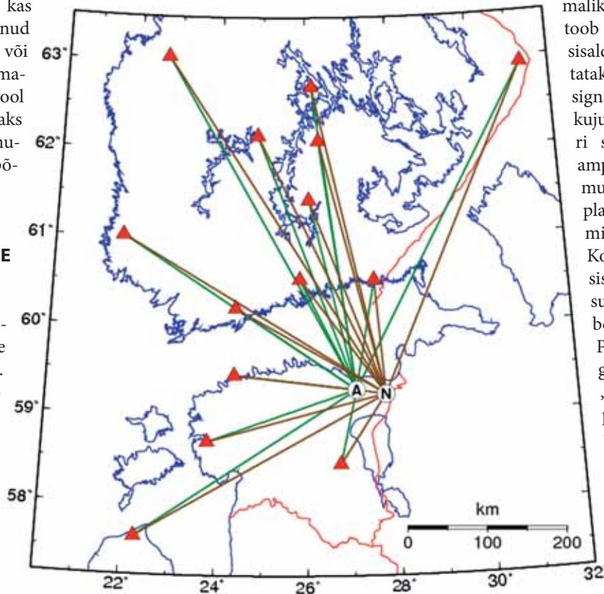
Joonis 1. Eesti seismojaamad ning meie seismoanalüüsis regulaarselt kasutatavad Soome ja Läti seismojaamad. Märkitud on Aidu (A) ja Narva (N) karjääri asukohad seismovõrgu suhtes. Üldjuhul rahuldava lokaliseeringu tingimuse kohaselt asuvad sündmused võrgu sees, s.t kõige suurem kahe jaama vaheline nurk on <180. Aidu puhul on see tingimus täidetud, aga Narva puhul mitte päriselt.
