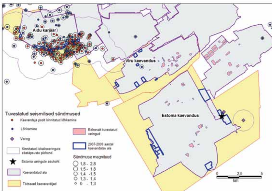
Joonis 2. Põlevkivimaardla alalt lokaliseeritud seismilised sündmused (lõhkamised ja varingud) jaanuaris ja oktoobris 2008
